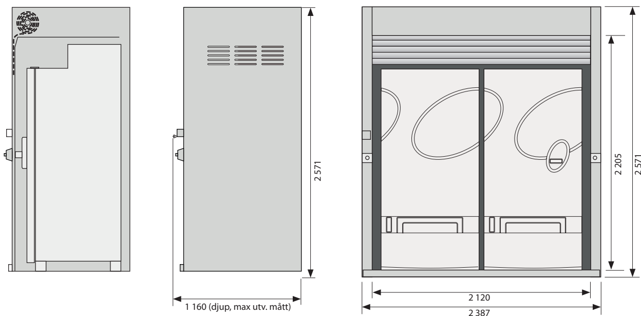
Utvändiga/invändiga mått, exempel V2
